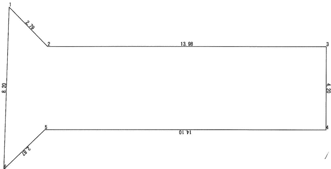
道路求積図
