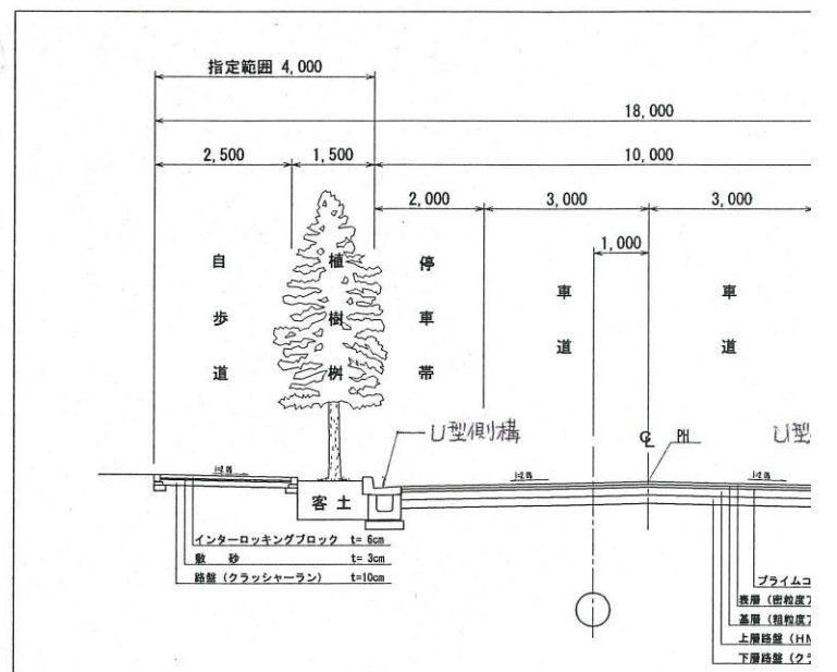
B-B断面
