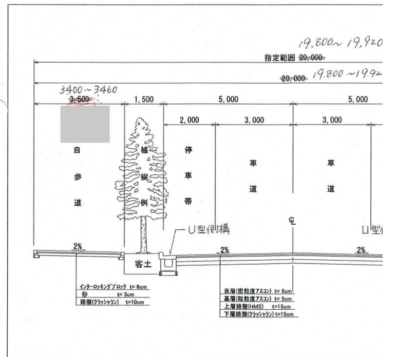
B-B断面
