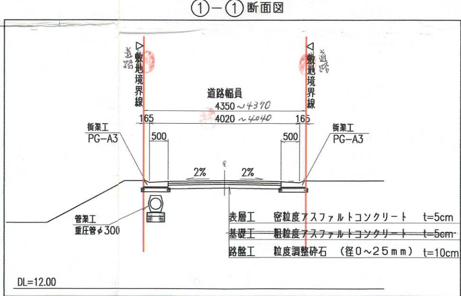
道路横断面図 S=1:100
