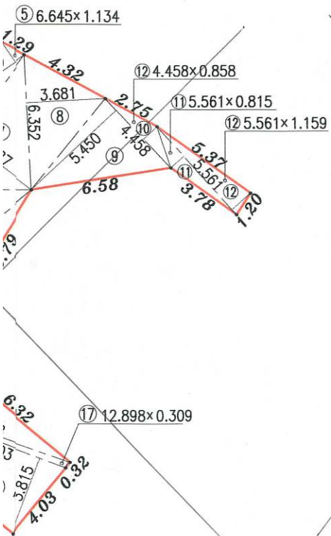
求積図 S=1:250
