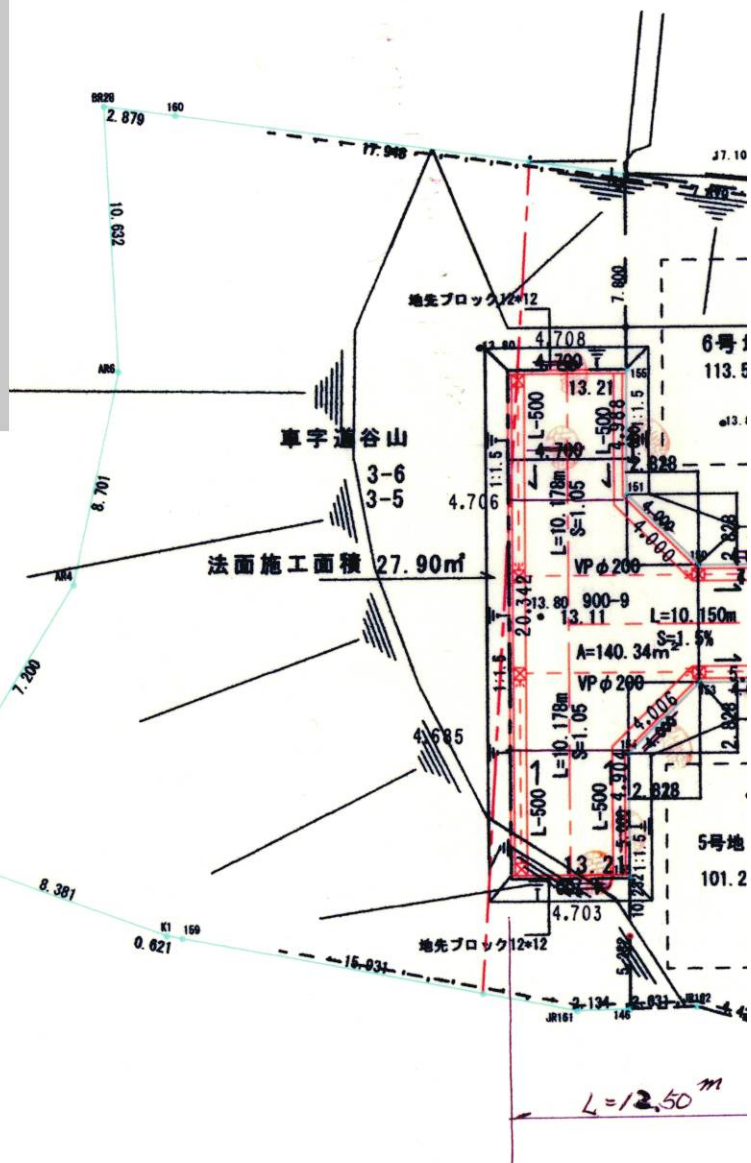
道路図(平面図)
