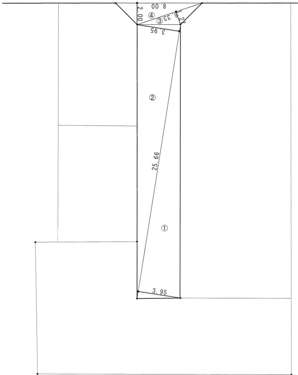
道路面積求積表
