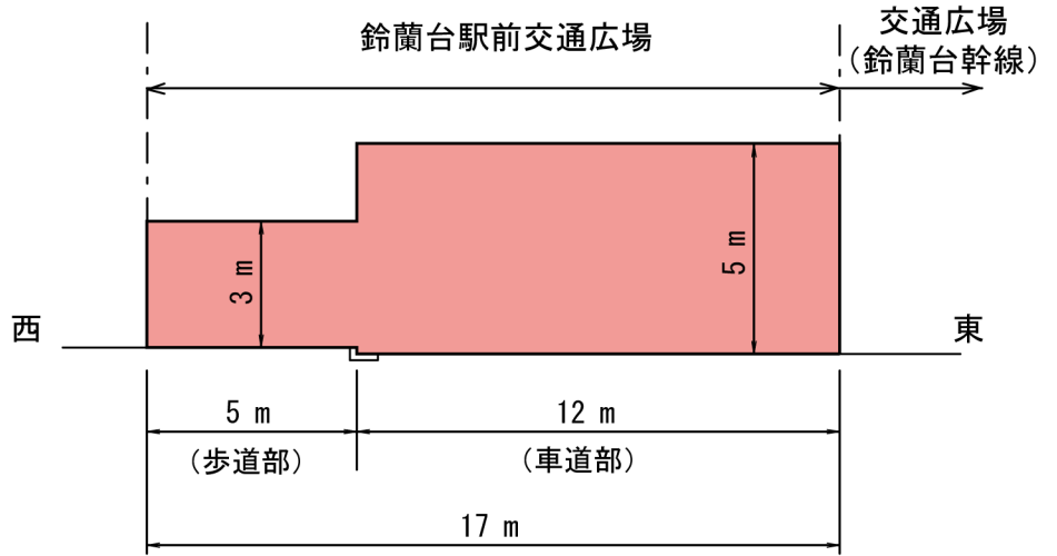
A-A' 断面
