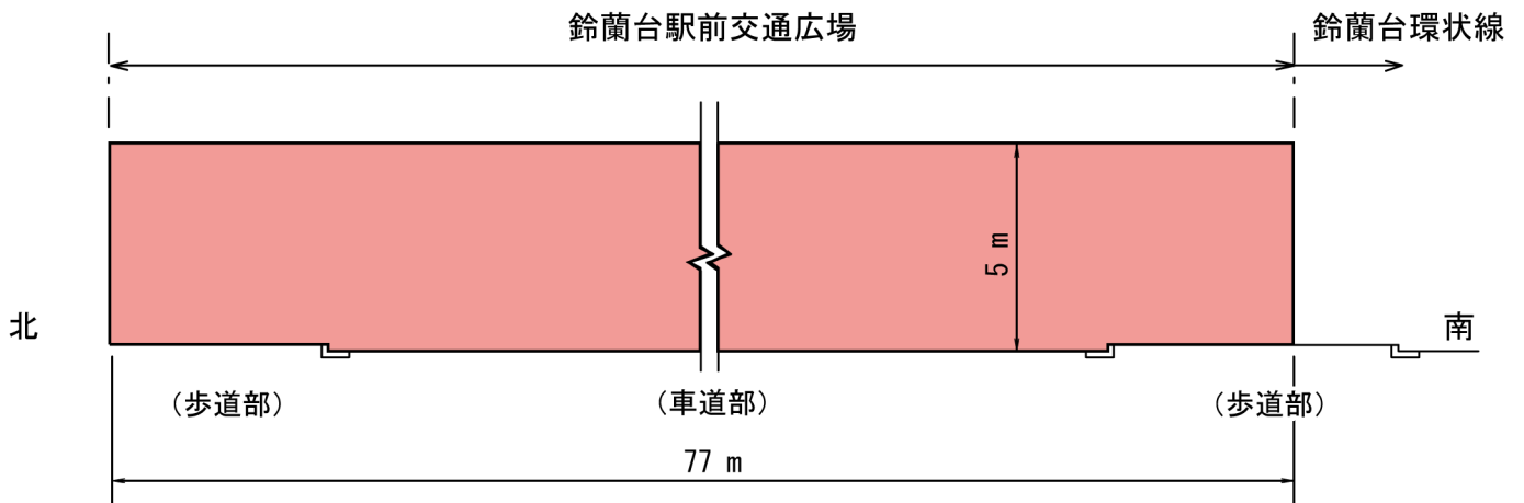
B-B' 断面
